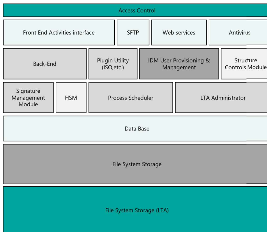
Componenti del Sistema di conservazione
